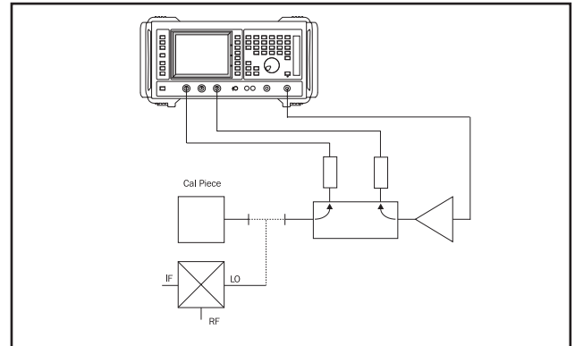
Fig. 9 LO Port Return Loss
